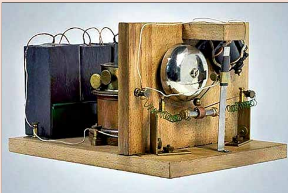
Прибор для обнаружения и регистрирования электрических колебаний А. Попова
